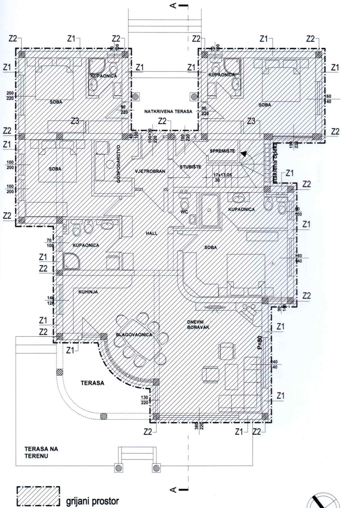
TLOCRT PRIZEMLJA
