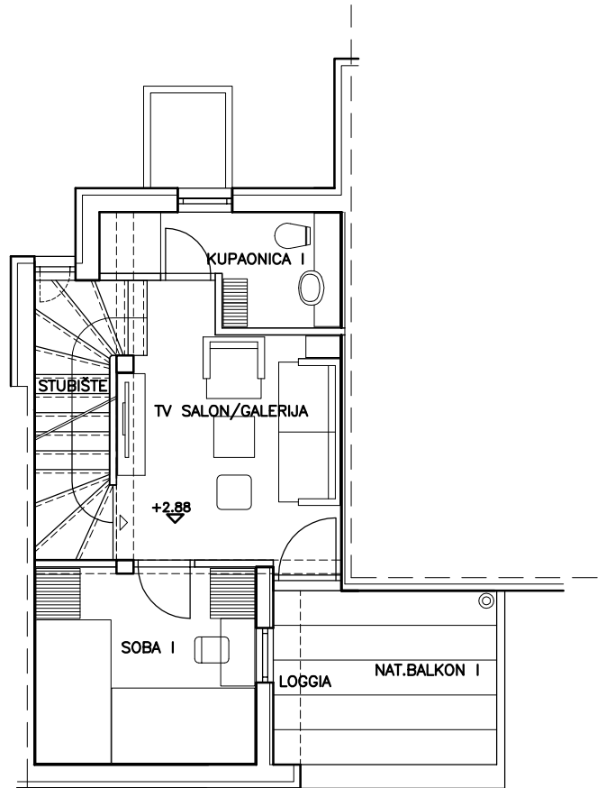
TLOCRT I.KATA
