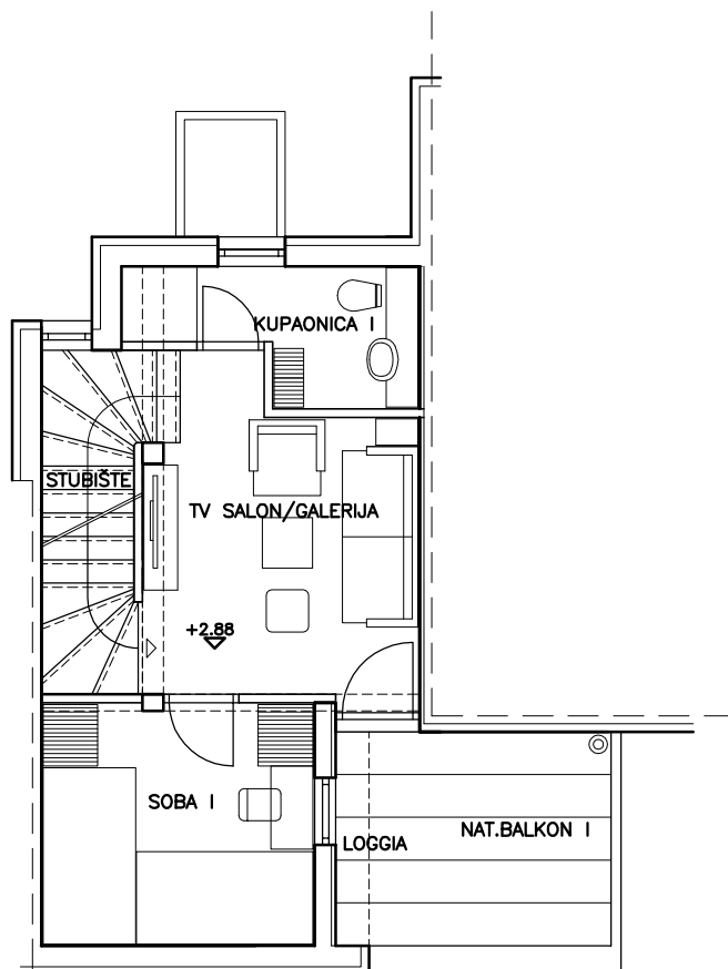
TLOCRT I.KATA
