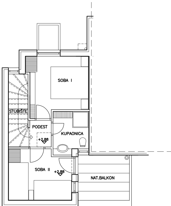
TLOCRT I.KATA
