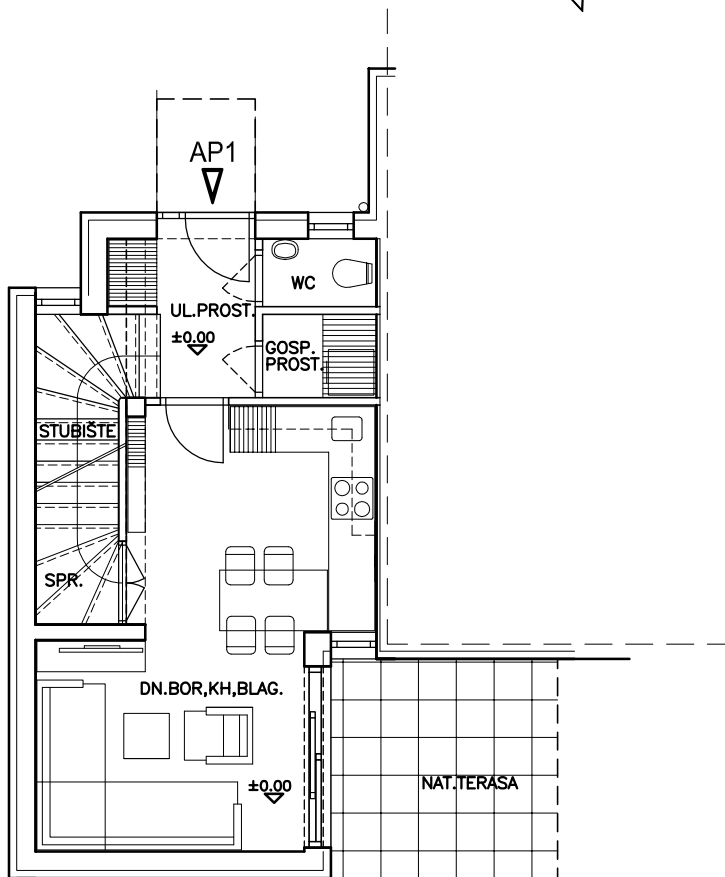
TLOCRT PRIZEMLJA
